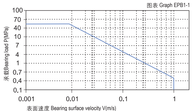
■ PV图表 Permissible PV value for CSB-EPB1
